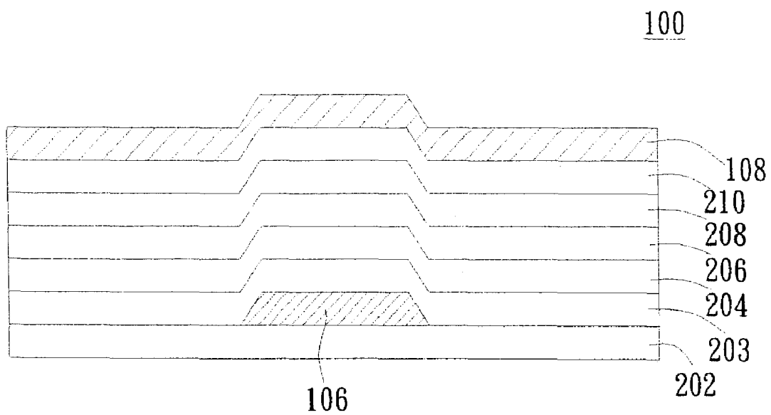
FIG. 3B(PRIOR ART)
